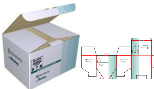
ящик со складным дном «ласточкин хвост»
