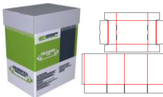
ящик крышка - дно
